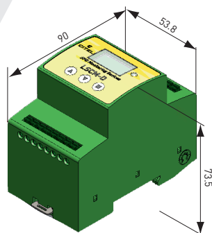
Устройство для мониторинга УЗИПов LSCM-D/24
