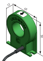
Сенсор LSCM-P1000
