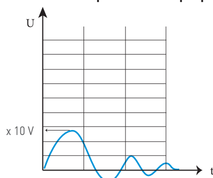
Четвертьволновой разрядник
