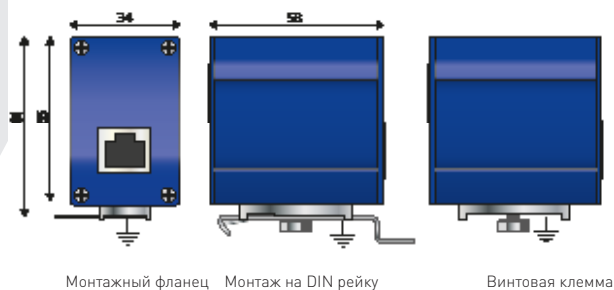
Монтажный фланец
