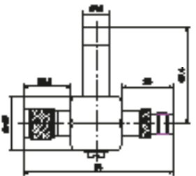
ПЧД105-Т/МФ
